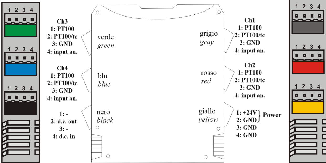
Fig 8: Morsettiere
